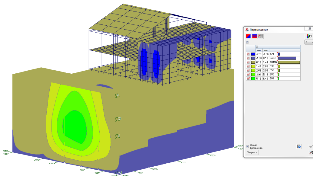
Рис. 4. Перемещения системы по направлению X при комбинации нагрузок.
