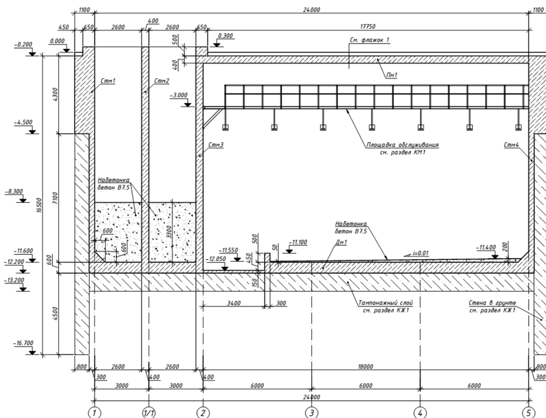
Рис. 1. Заглубленный ж/б резервуар. Разрез.
