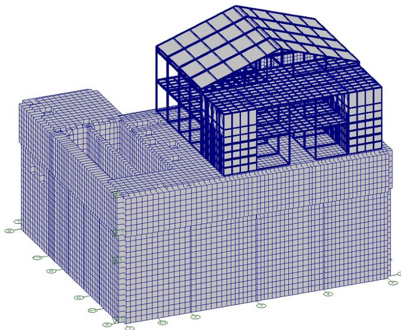
Рис.3. Общий вид расчетной модели.
